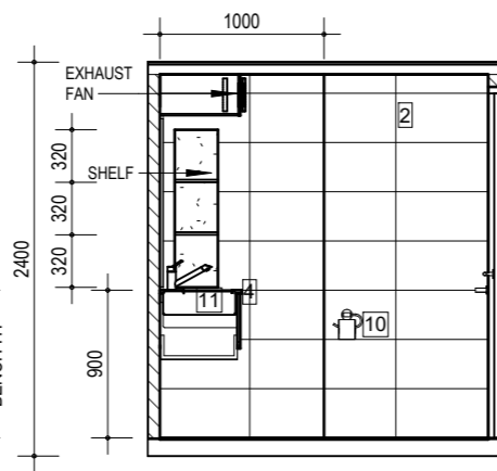
ELEVATION 2
