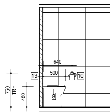
ELEVATION 8
