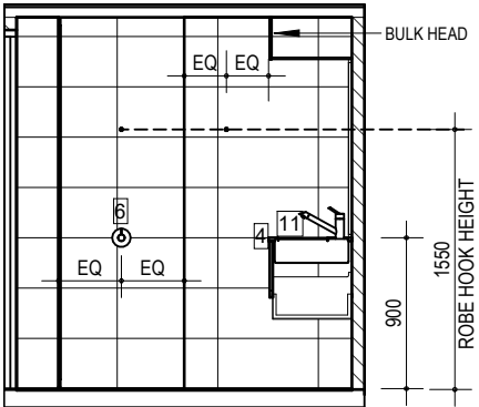
ELEVATION 4 1 : 50
