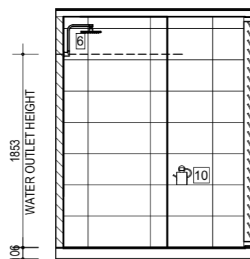
ELEVATION 6
