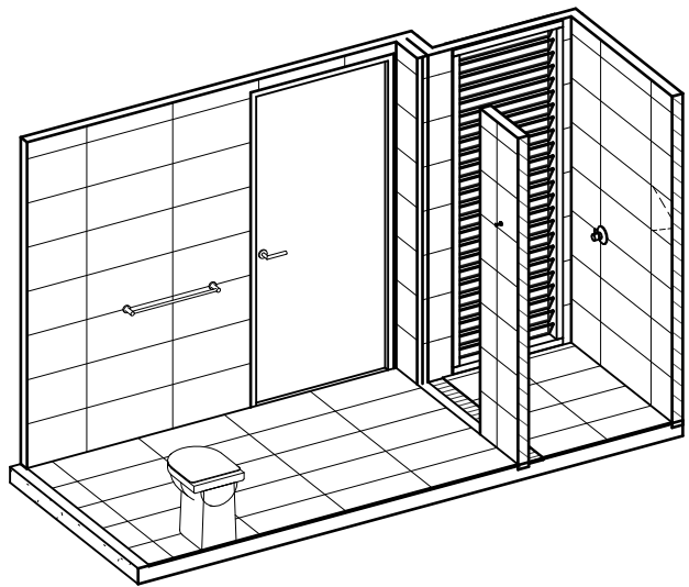
BACK AXO
