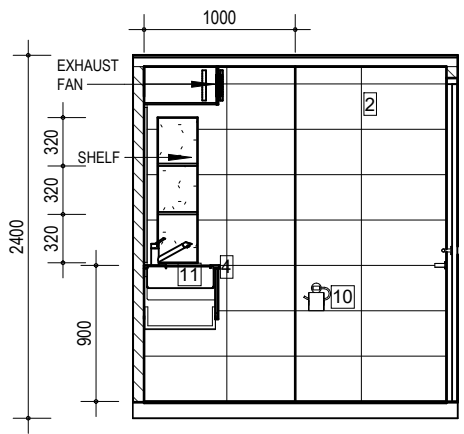
ELEVATION 2 1 : 50
