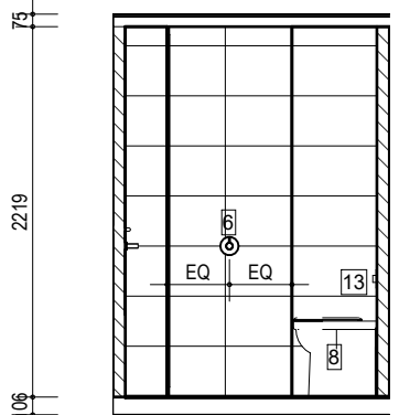
ELEVATION 7 1 : 50
