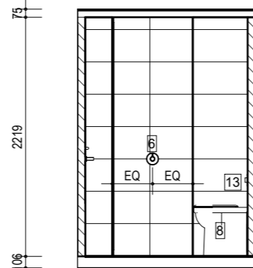
ELEVATION 7
