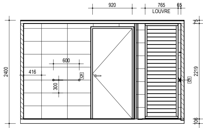
ELEVATION 3 1 : 50
