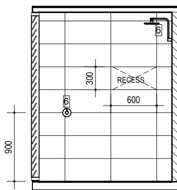
ELEVATION 5 1 : 50
