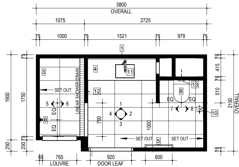
FLOOR PLAN 1 : 50
