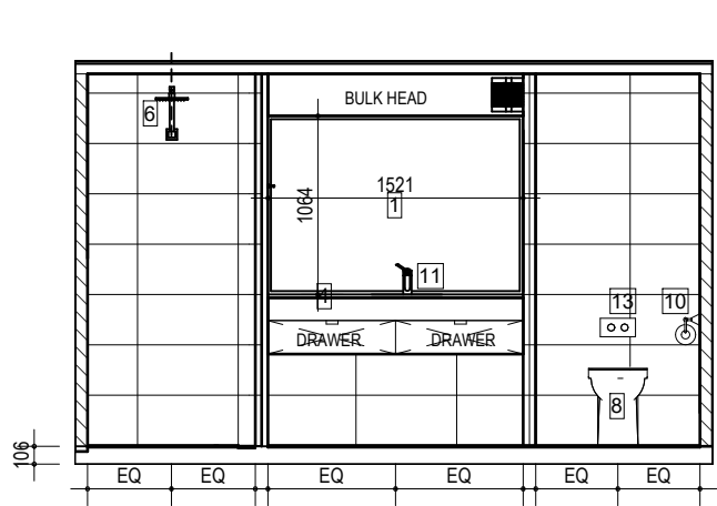
ELEVATION 1 1 : 50
