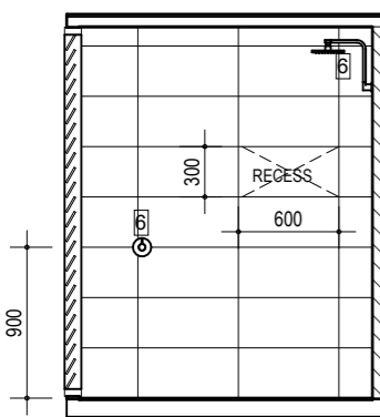
ELEVATION 5
