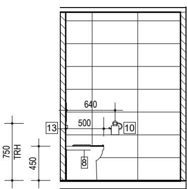
ELEVATION 8 1 : 50
