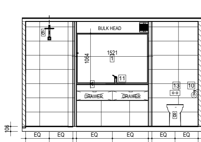
ELEVATION 1
