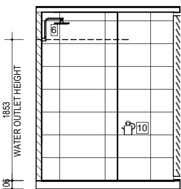
ELEVATION 6 1 : 50
