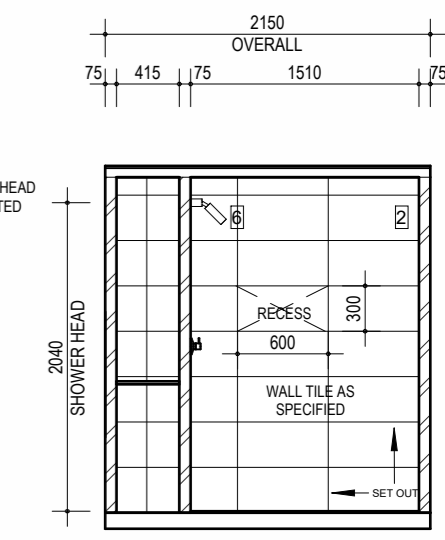
ELEVATION 5 1 : 50
