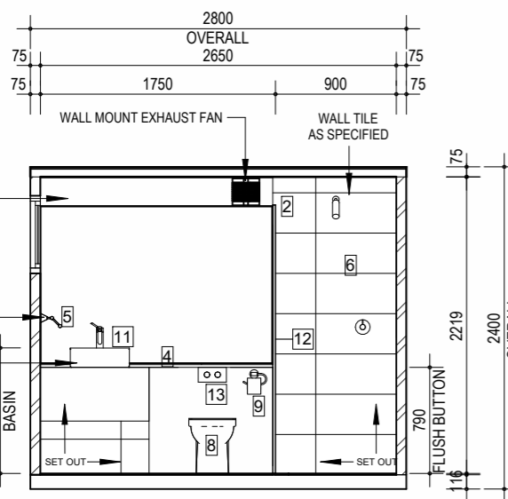
ELEVATION 1 1 : 50
