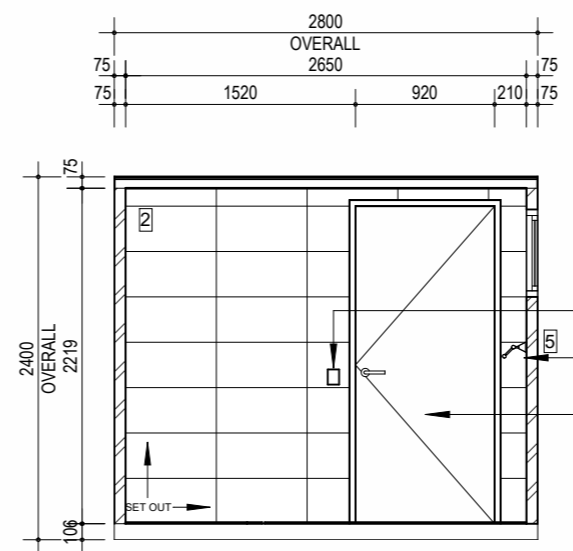
ELEVATION 3 1 : 50
