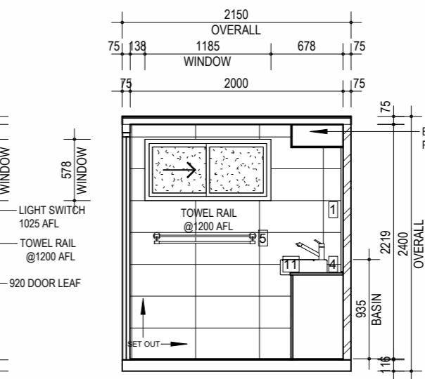
ELEVATION 4 1 : 50
