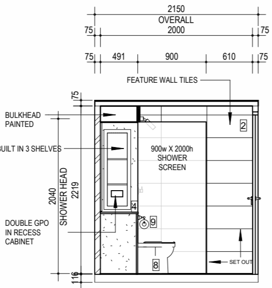
ELEVATION 2 1 : 50
