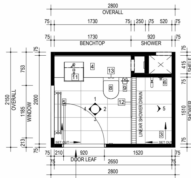
FLOOR PLAN 1 : 50
